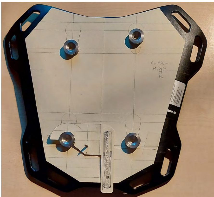
Halterung - Diebstahlsicherung die von unten verbaut wird, und mit einem Vorhängeschloss gesichert. Die Platte wird an den originalen Bohrungen mit 10mm Abstand zum Rack verschraubt, benötigt für den Riegel.
